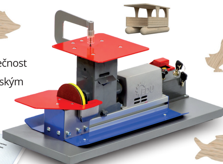
EDUpilka s čelní bruskou
